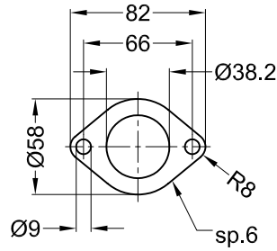
Vista "B" Flangia "23D"
