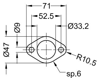
Vista "B" Flangia "43A"
